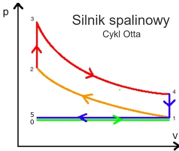
Cykl Otto
