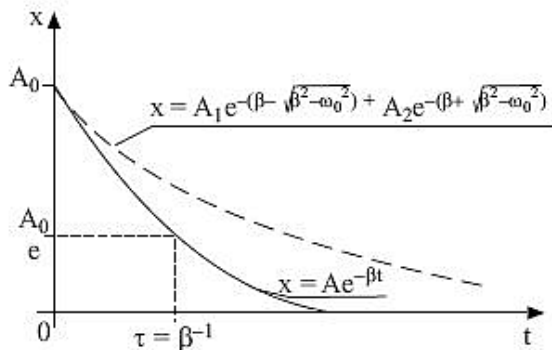
Zależności x = x(t) dla dwóch rozwiązań aperiodycznych \beta = \omega_o i \beta > \omega_o
